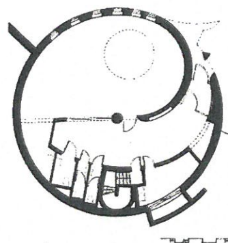
Obr.č. 5. Stavba svým měřítkem vychází z pražské kaple sv. Václava – kruhem opisuje její čtvercový půdorys. Půdorys přízemí – 1 n.p. / VIZUALIZACE
